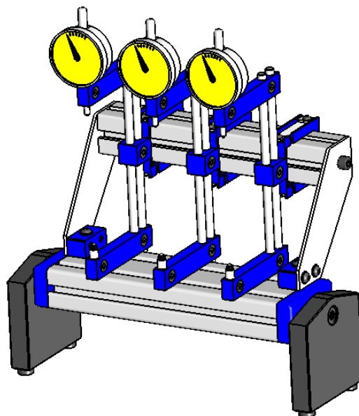
MD-5037 Spitzenhöhe 100mm mit Rachenlehre MD-5035-2
