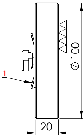
Messplatte KM-1017-0 gehärtet-geschliffen
