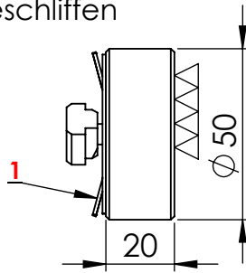
Messplatte KM-1017-0 gehärtet-geschliffen
