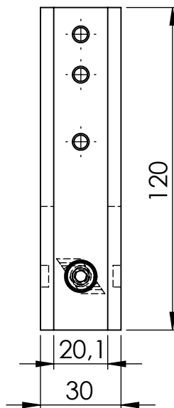
Verlängerung KM-1010-0 (-1) für Universalschwenkarm MD-3010 Bestellnummer - 0 = Aluminium blau-eloxiert - 1 = Stahl matt-vernickelt
