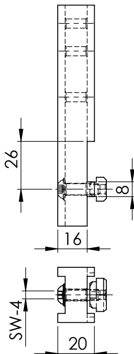
Verlängerung KM-1010-0 (-1) für Universalschwenkarm MD-3010 Bestellnummer - 0 = Aluminium blau-eloxiert - 1 = Stahl matt-vernickelt
